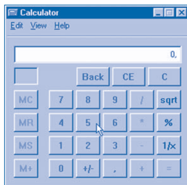
Fig. 3.4. Aplicația Calculator
