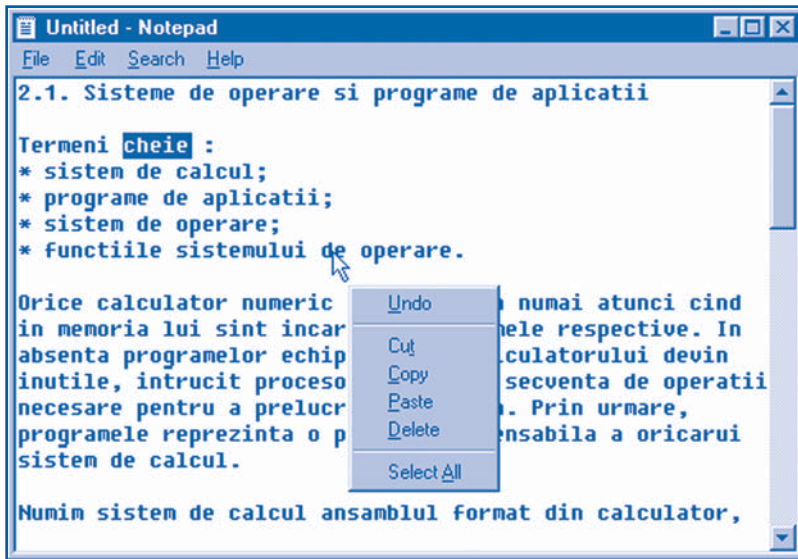
Fig. 3.8. Meniu contextual
