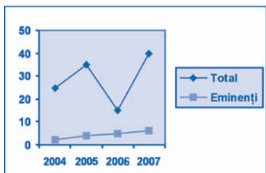
Diagramă liniară
