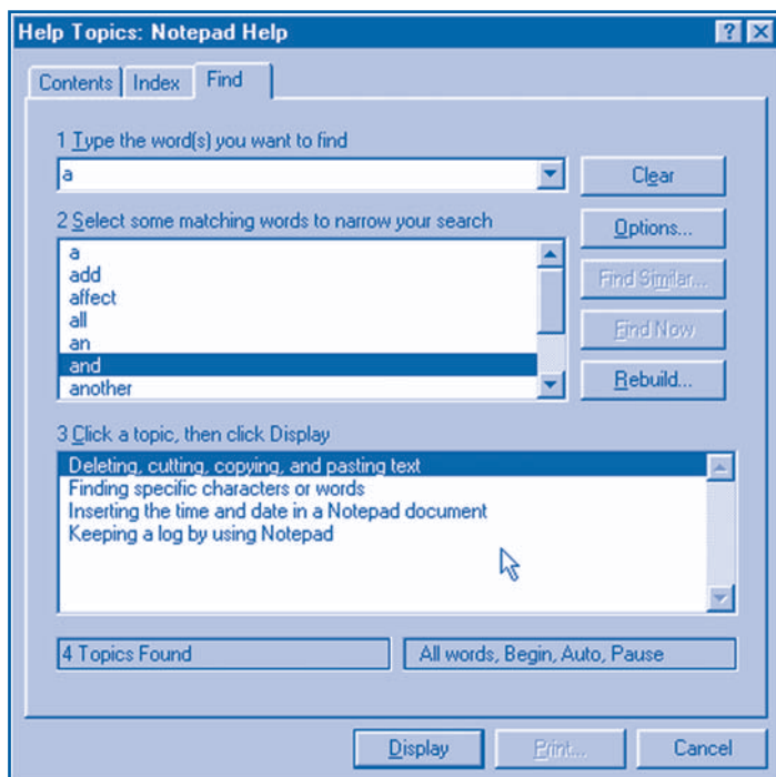
Fig. 3.20. Pagina Find
