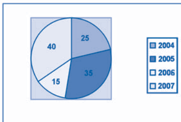
Diagramă circulară
